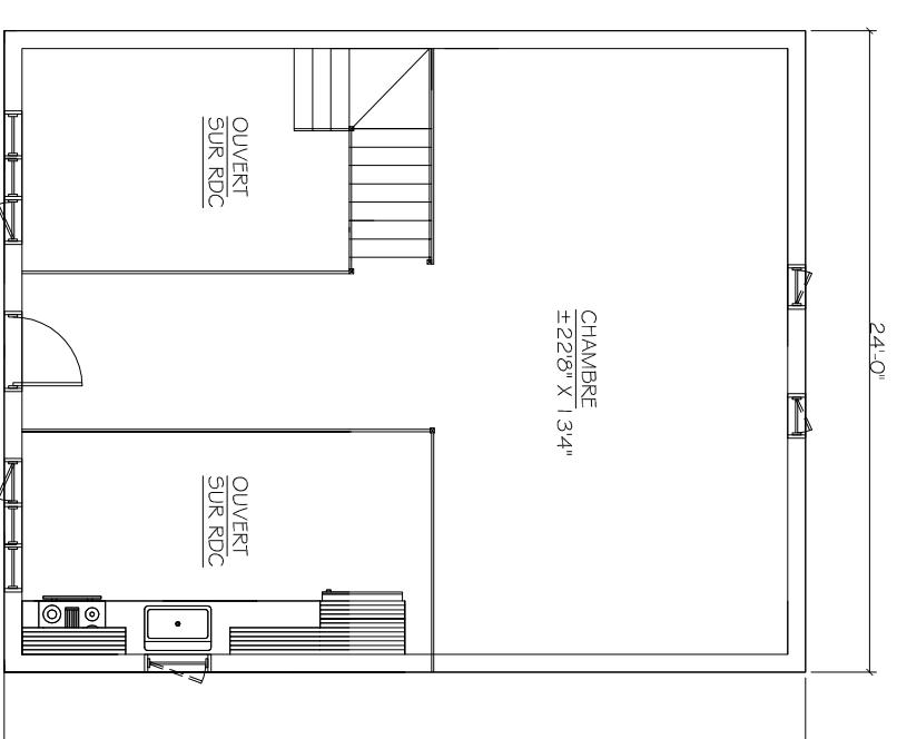
VUE ÉTAGE
