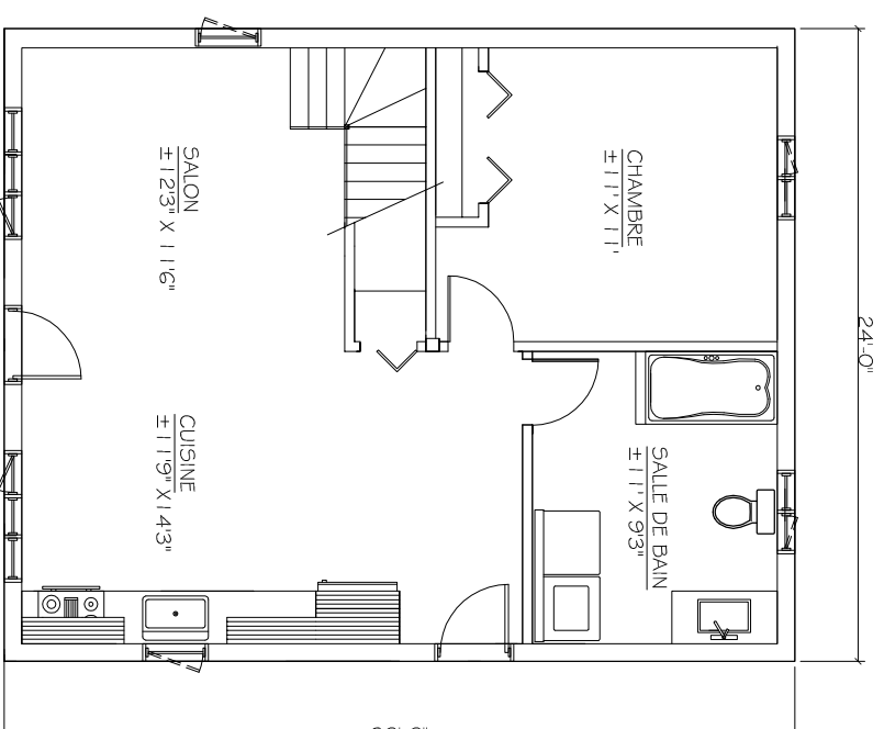
VUE RDC
